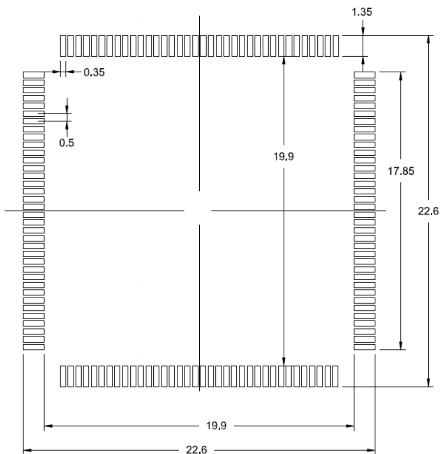
图 15 LQFP144-144 引脚，20 x 20 mm 焊接 Layout 建议
