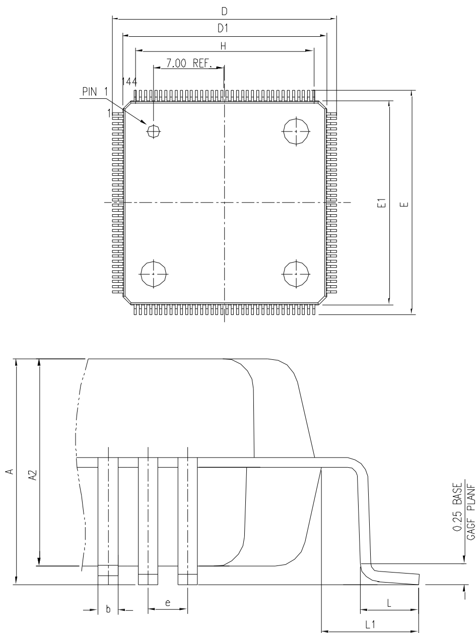
图 14 LQFP144 封装图
