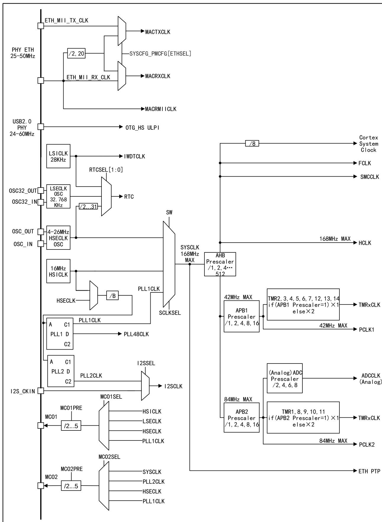
图 4 APM32A407xGT7 时钟树
