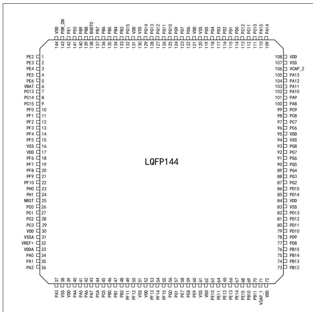
图 1 APM32A407xGT7 系列 LQFP144 引脚分布图
