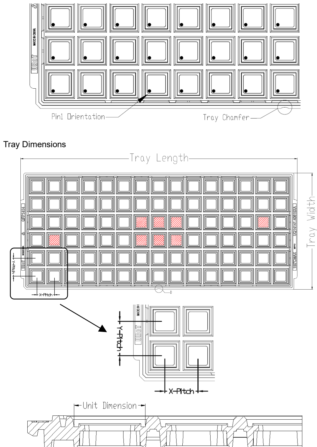
图 19 托盘包装示意图
