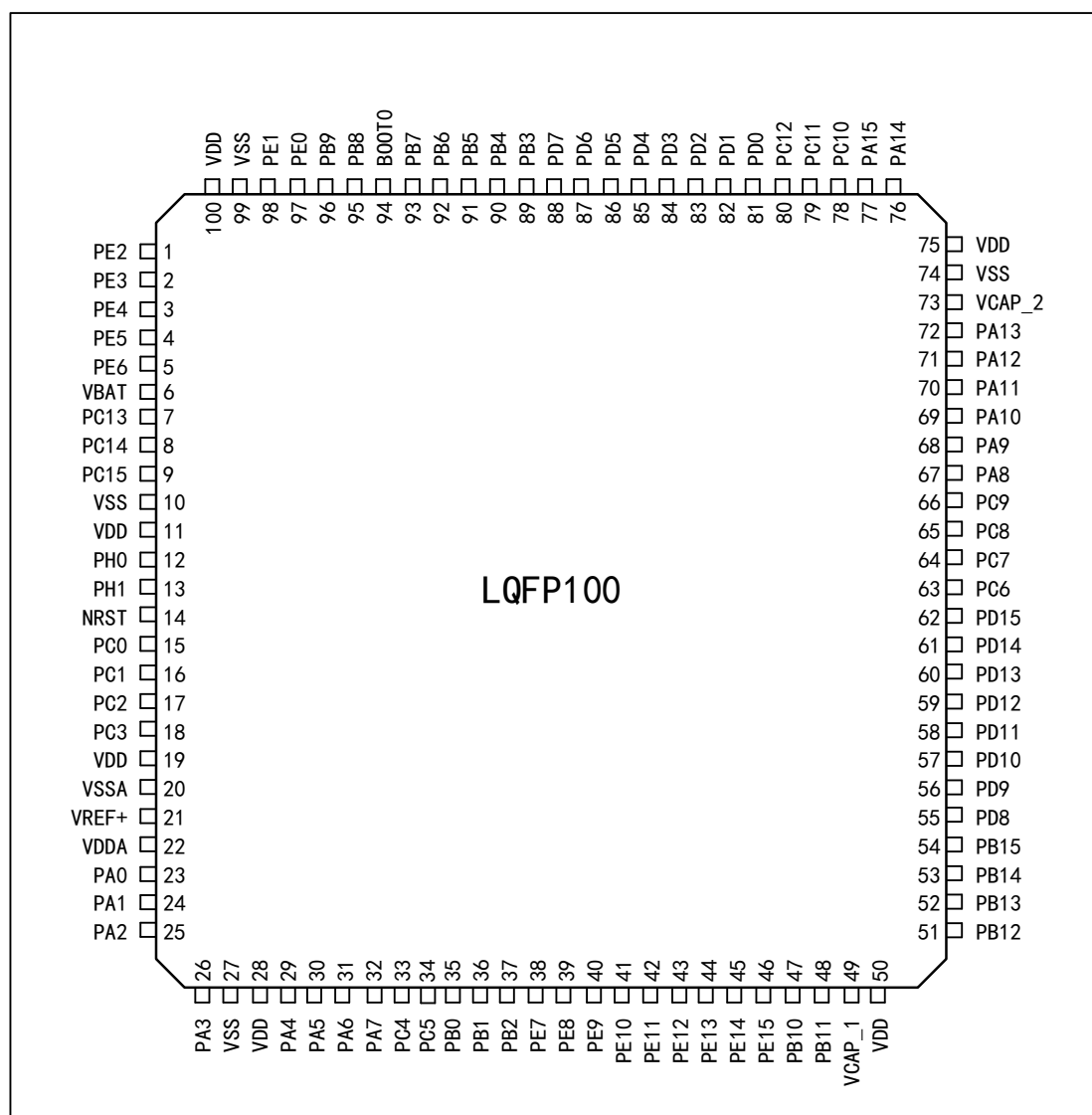
图 2 APM32A407xGT7 系列 LQFP100 引脚分布图
