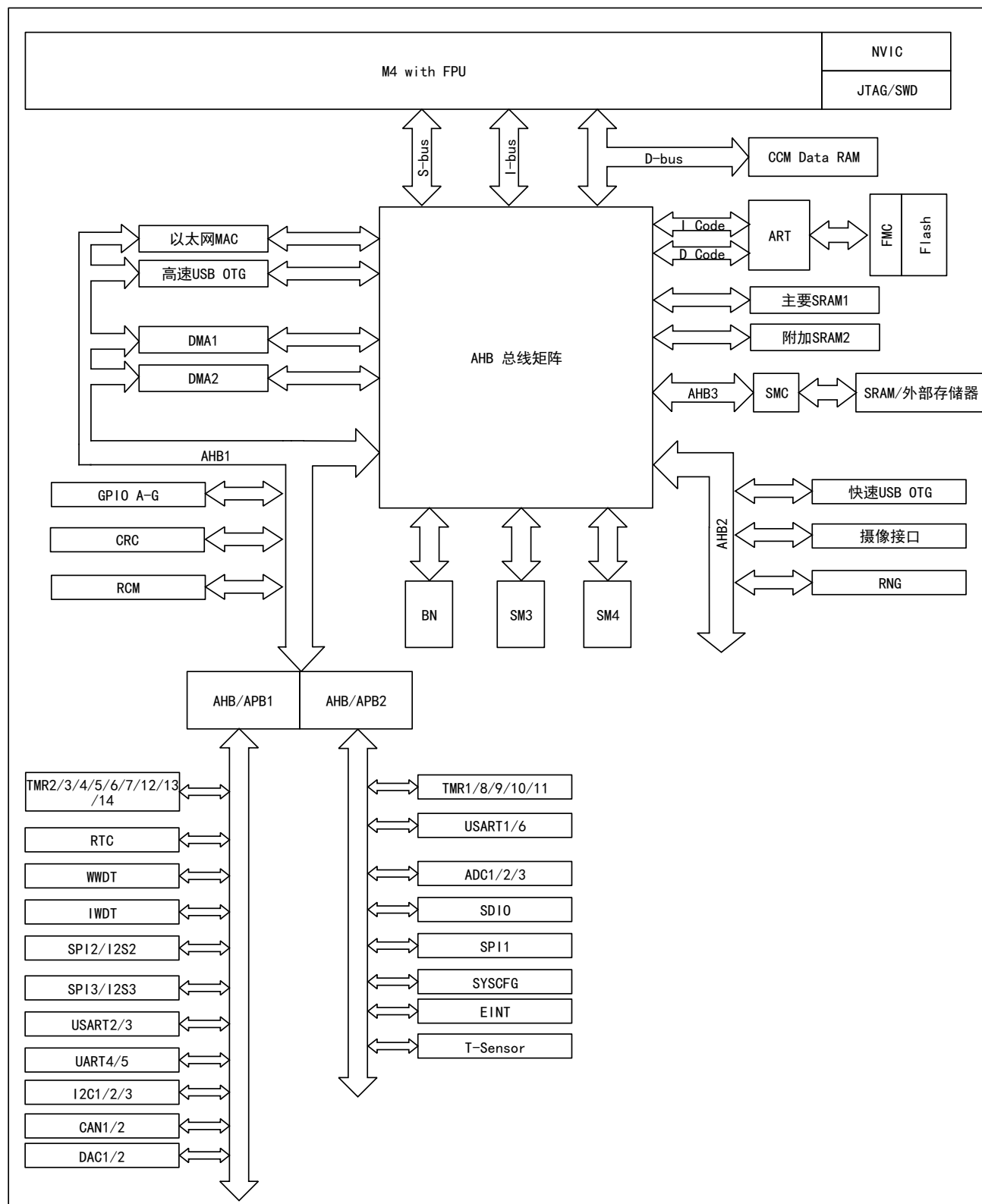
图 3 APM32A407xGT7 系统框图
