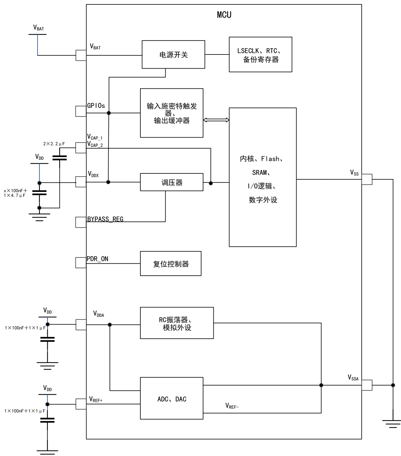
图 5 电源方案
